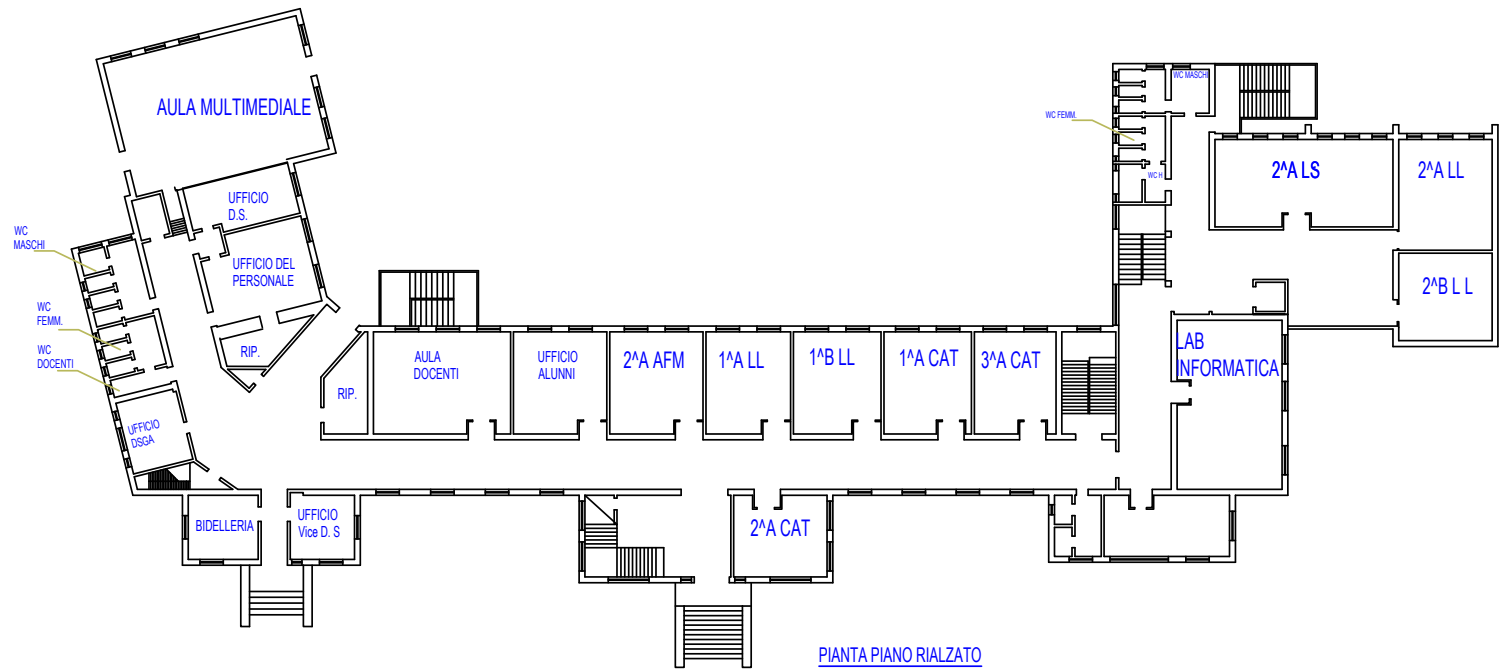
PIANTA PIANO RIALZATO
